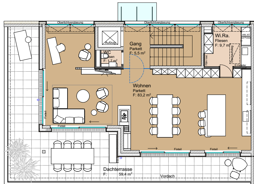
OBERGESCHOSS M 1:100
