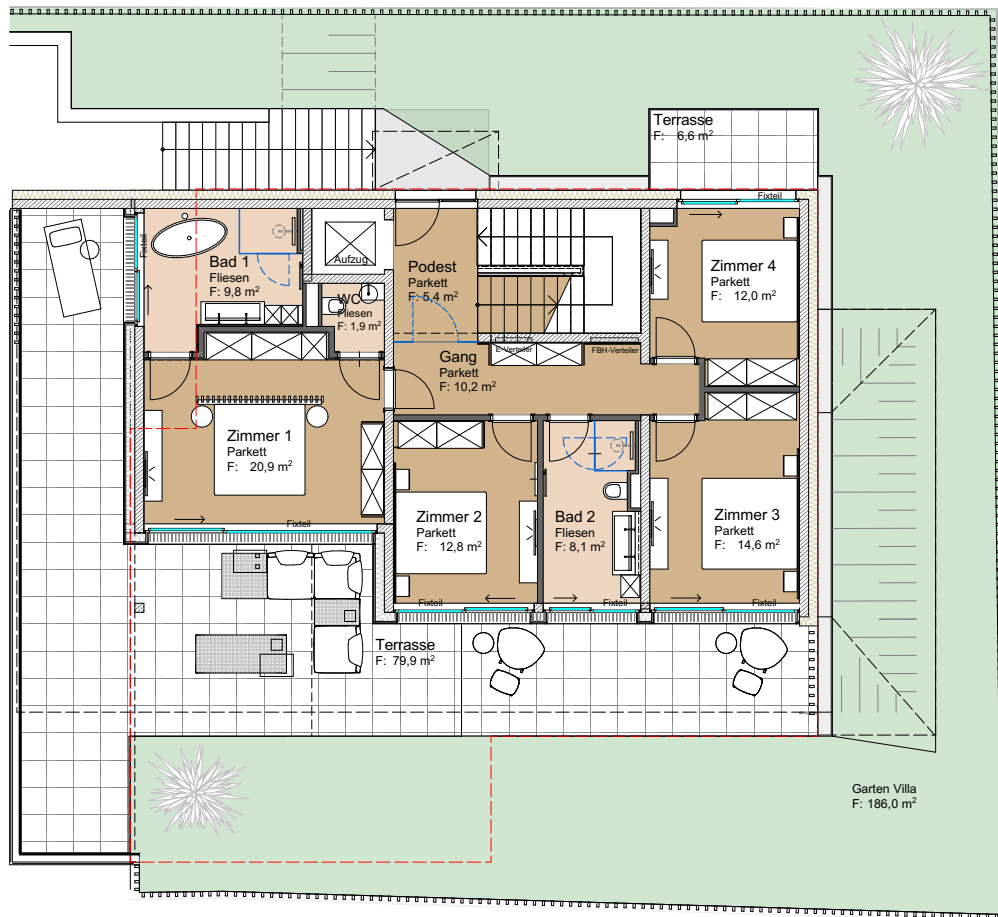
ERDGESCHOSS M 1:100
