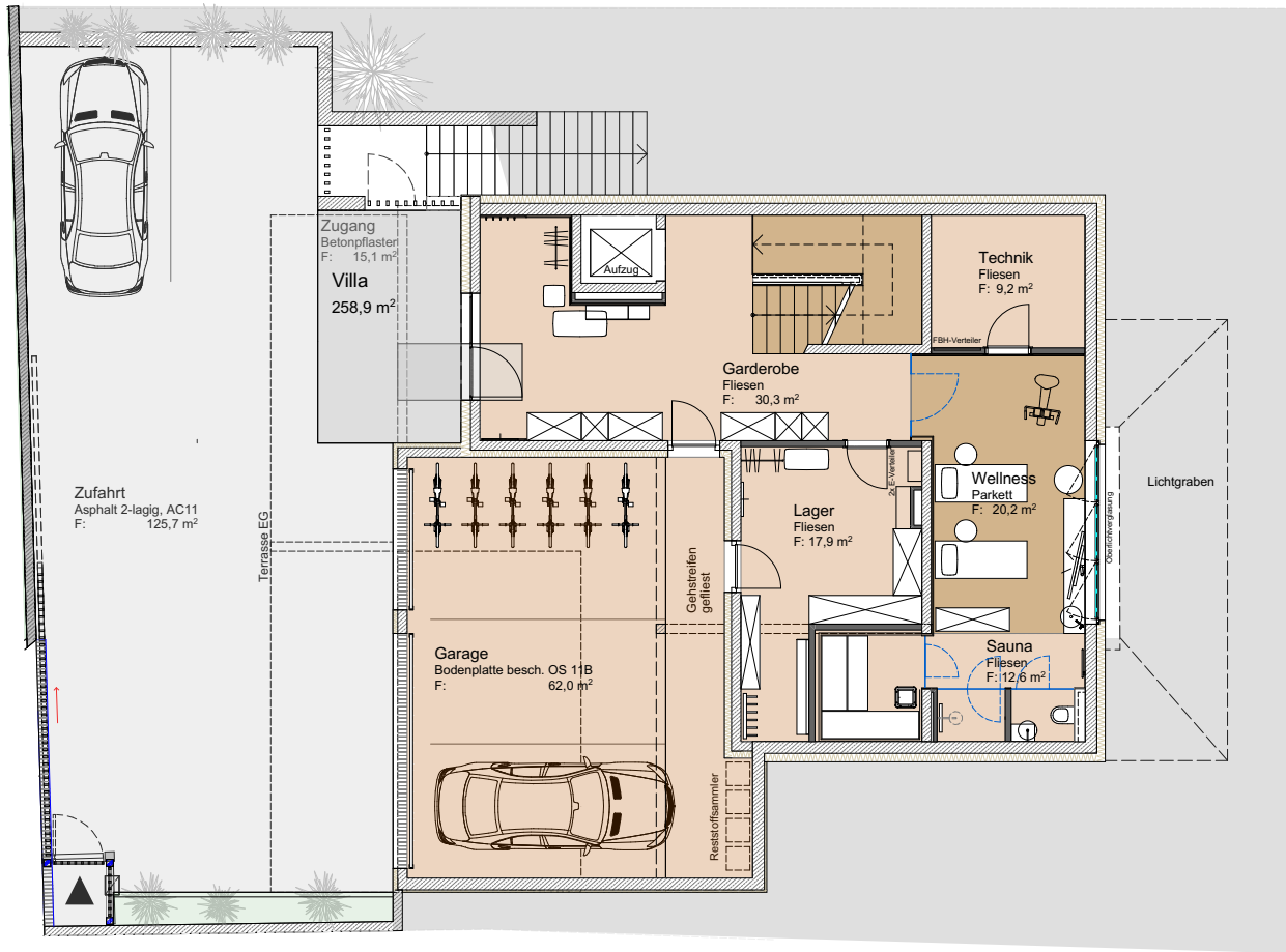
UNTERGESCHOSS M 1:100
